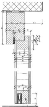
Schnitt B-B Mst. 1:1
