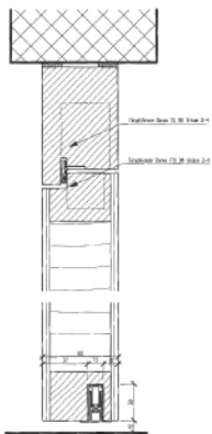
Schnitt B-B Mst. 1:1
