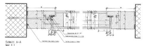
Schnitt A-A Mst. 1:1
